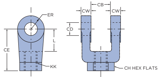
ROD CLEVIS
