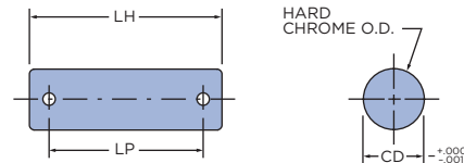
ROD EYE
